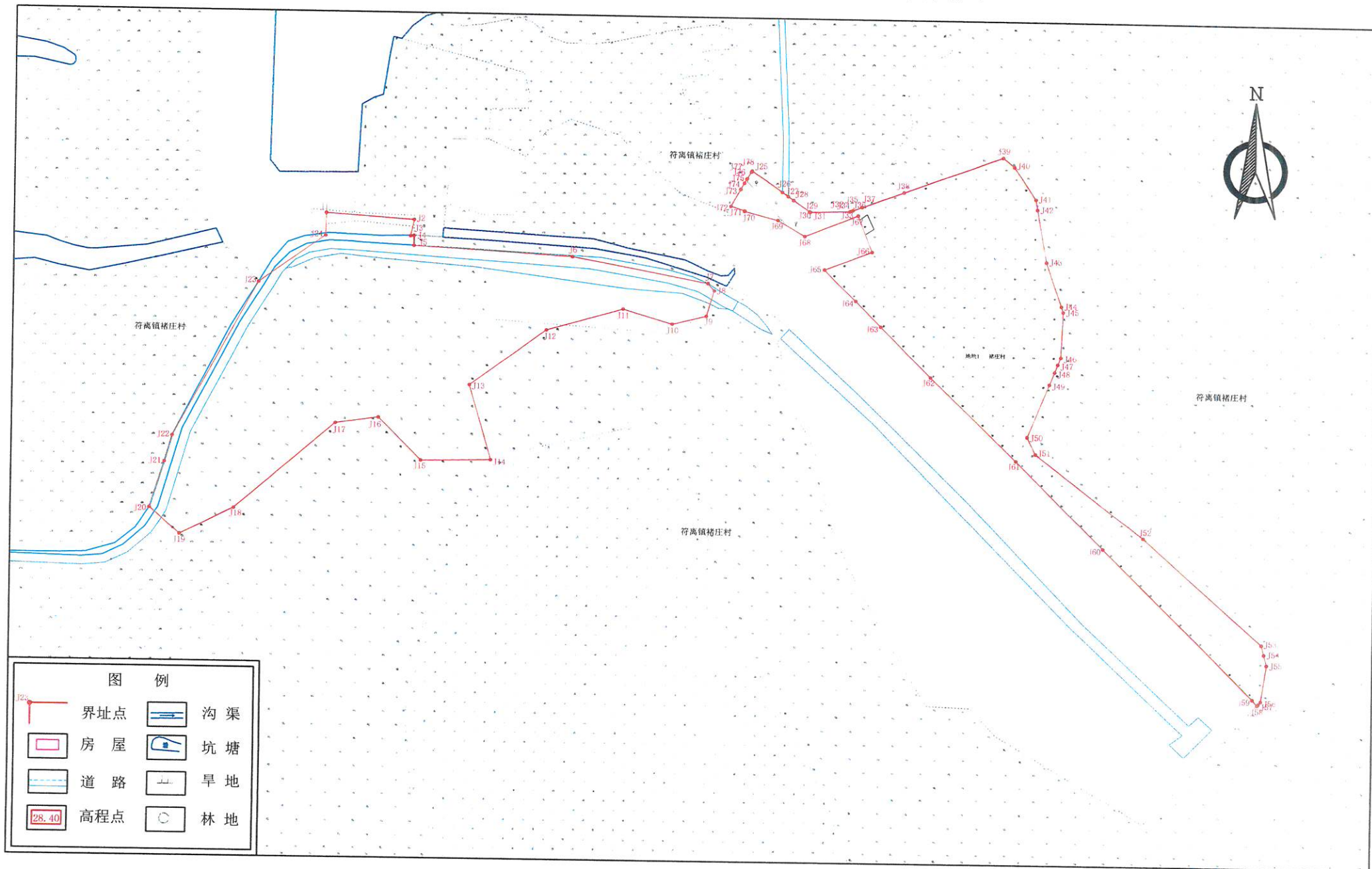
埇桥区城市公益性公墓（芦村）项目勘测定界简图
