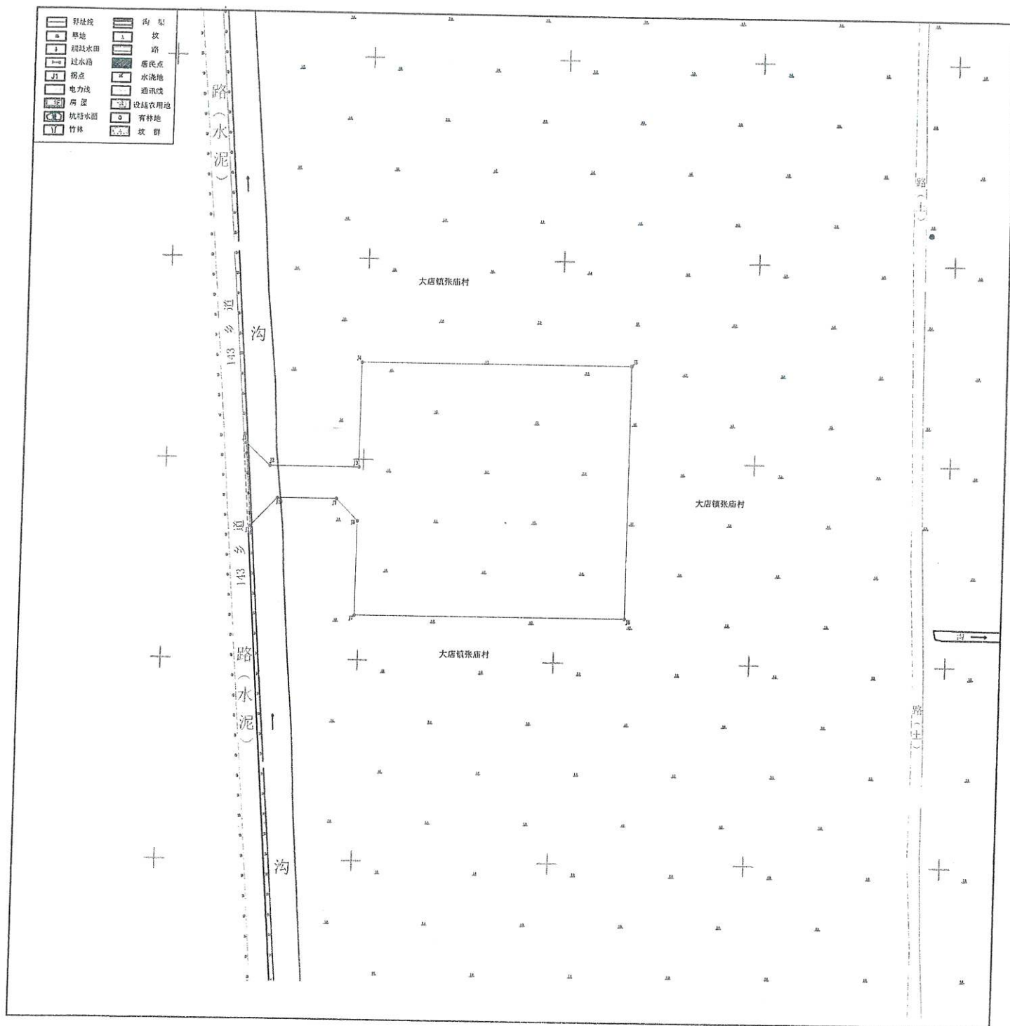
安徽宿州土楼110kV输变电工程勘测定界简图
