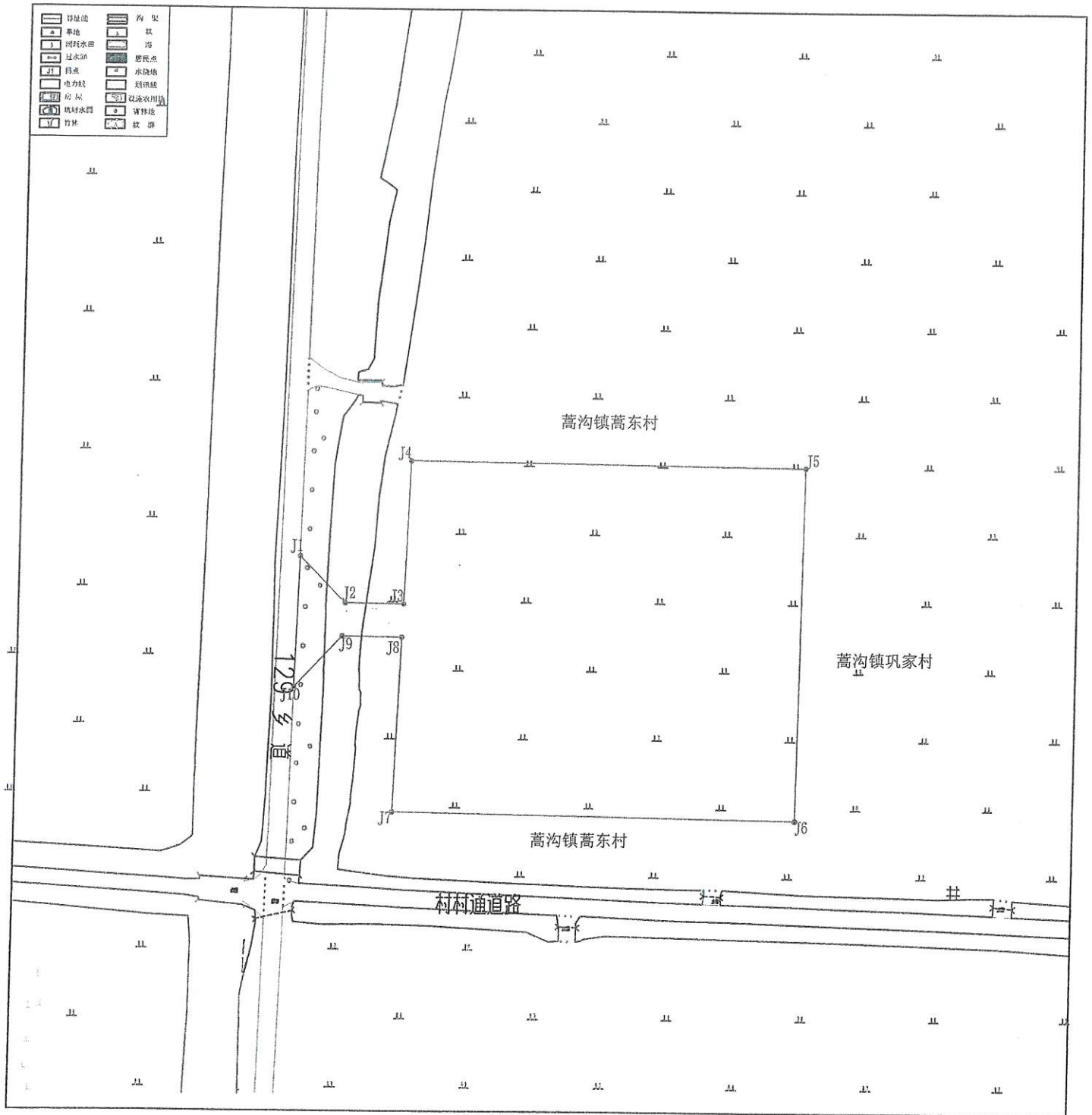
安徽宿州宿马220kV输变电工程勘测定界简图
