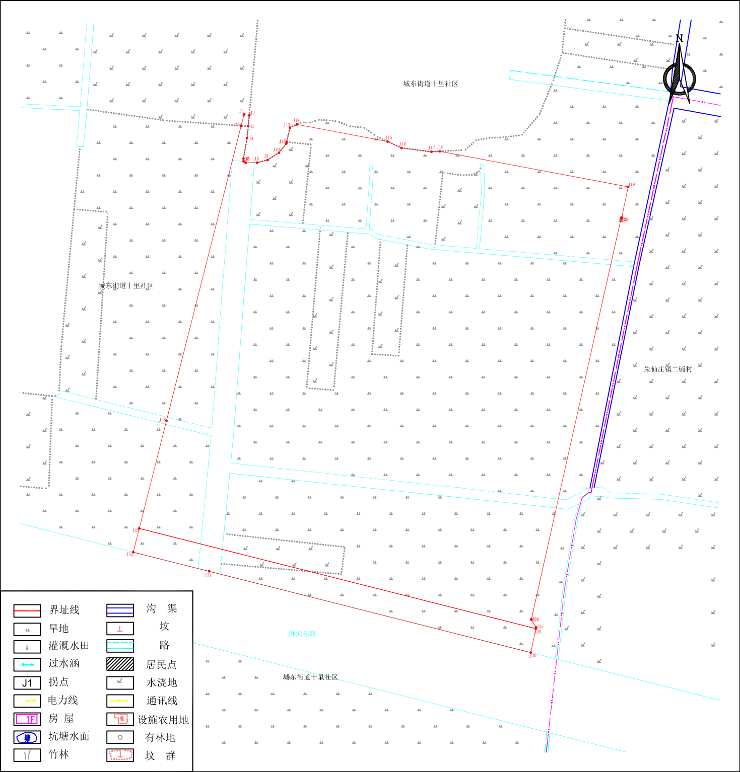
宿州市埇桥区2024年第3批次（增减挂钩）城镇建设用地勘测定界简图
