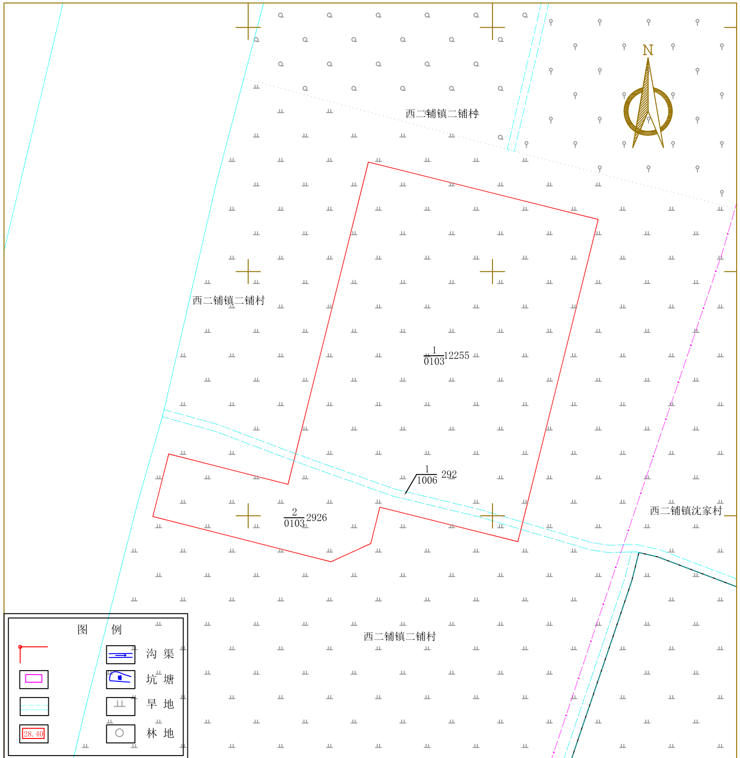
宿州城西220千伏输变电工程项目勘测定界简图
